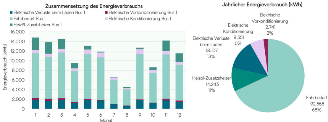
Abbildung 51: Ausbaustufe 1 - Zusammensetzung des Energieverbrauchs der Busse
