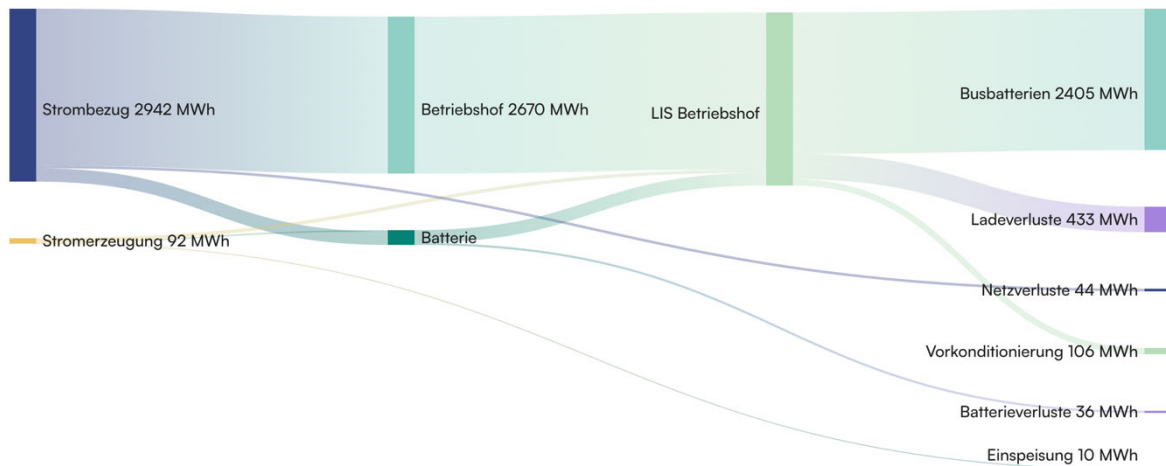
Abbildung 48: Elektrischer Energiefluss für Ausbaustufe 2 — Variante 4 mit PV-Anlage & Batteriespeicher
