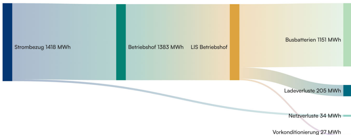
Abbildung 31: Elektrischer Energiefluss für Ausbaustufe 1 — Variante 1 mit reinem Strombezug
