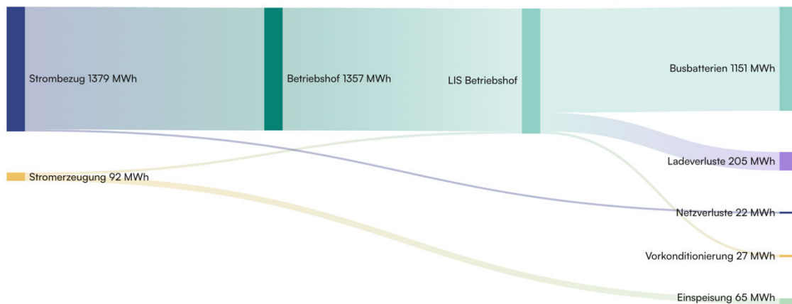
Abbildung 33: Elektrischer Energiefluss für Ausbaustufe 1 und Variante 3 mit PV-Anlage
