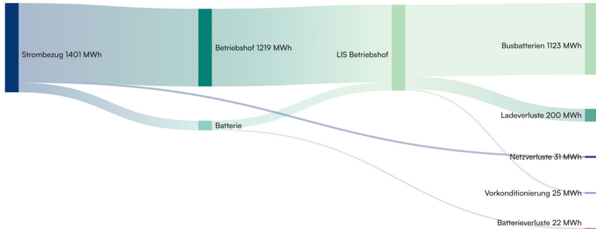
Abbildung 32: Elektrischer Energiefluss für Ausbaustufe 1 und Variante 2 mit Batterie
