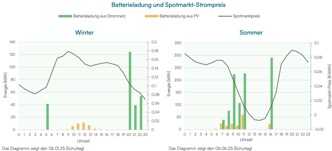
Abbildung 39: Batterieladung abhängig vom Spotmarkt-Strompreis in Variante 4 (Stufe 1)
