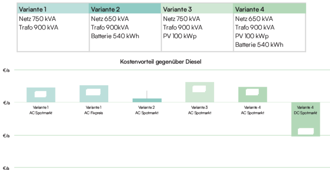
Abbildung 25: Kostenvorteil gegenüber Diesel (Stufe 1) — positiver Wert = Vorteil; negativer Wert = Nachteil
