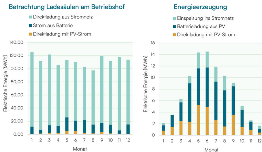
Abbildung 35: Monatlicher PV-Strom-Anteil am Energieverbrauch und Verhältnis von Eigennutzung und Einspeisung (Stufe 1)
