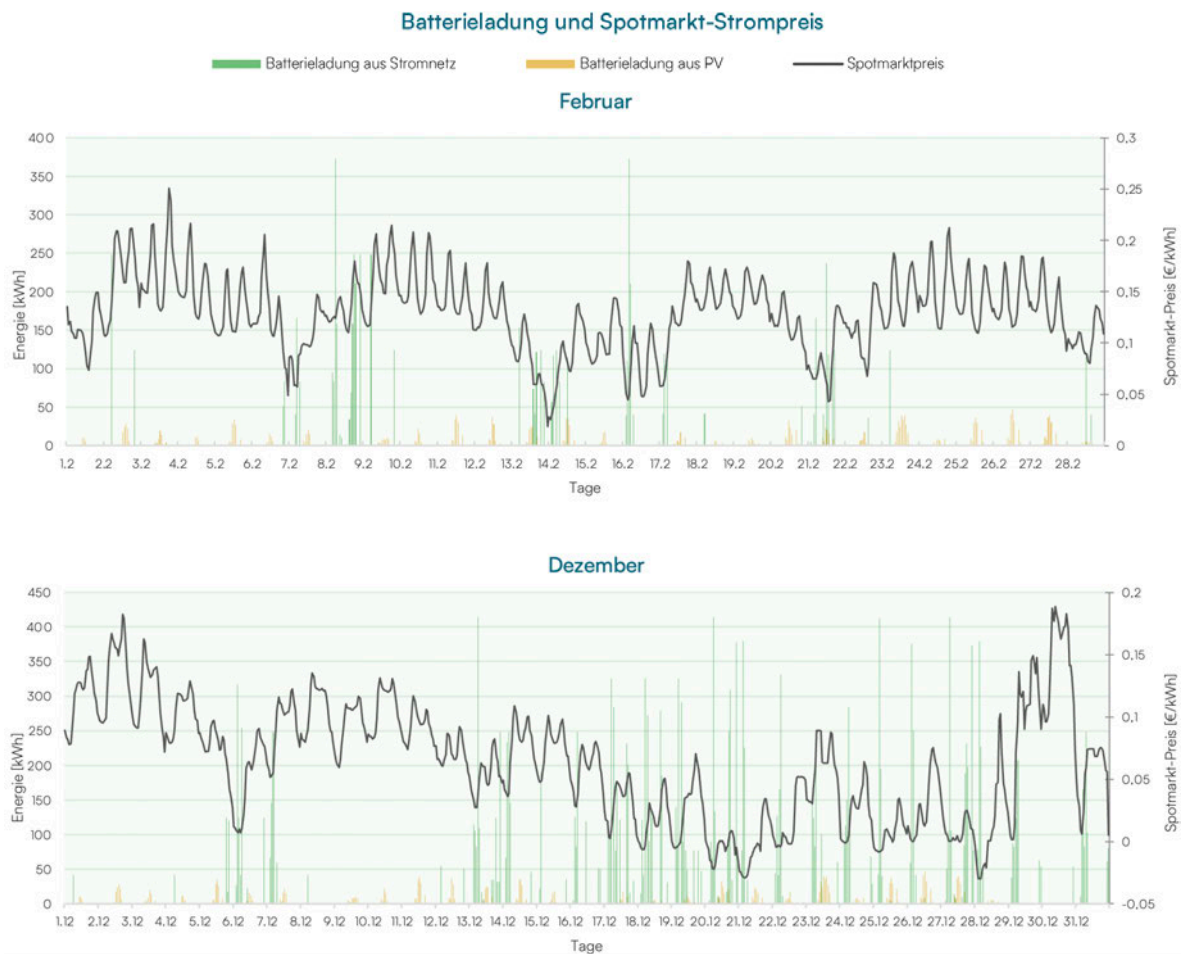
Abbildung 40: Ladezyklen der stationären Batterie im Februar und Dezember (Stufe 1 — Variante 4)
