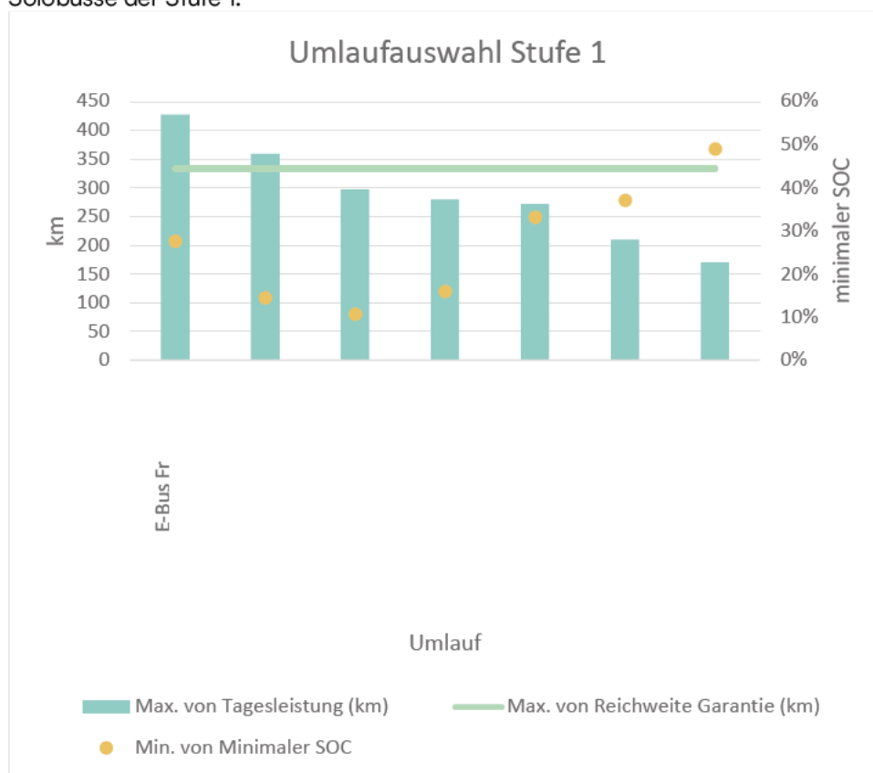
Abbildung 15: Solobusumläufe Stufe 1
