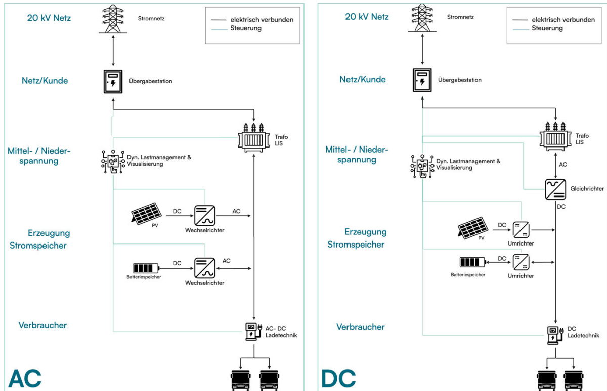
Abbildung 22: Schematische Darstellung des Energiesystems der Variante 4
