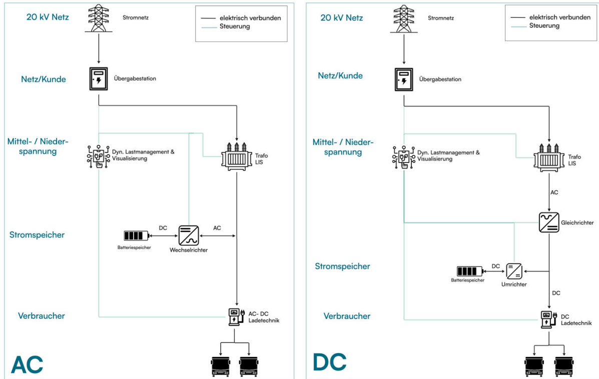
Abbildung 20: Schematische Darstellung des Energiesystems der Variante 2
