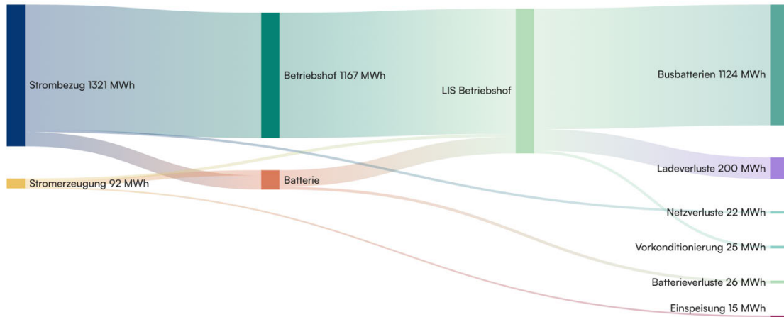
Abbildung 34: Elektrischer Energiefluss für Ausbaustufe 1 und Variante 4 mit PV-Anlage und Batterie
