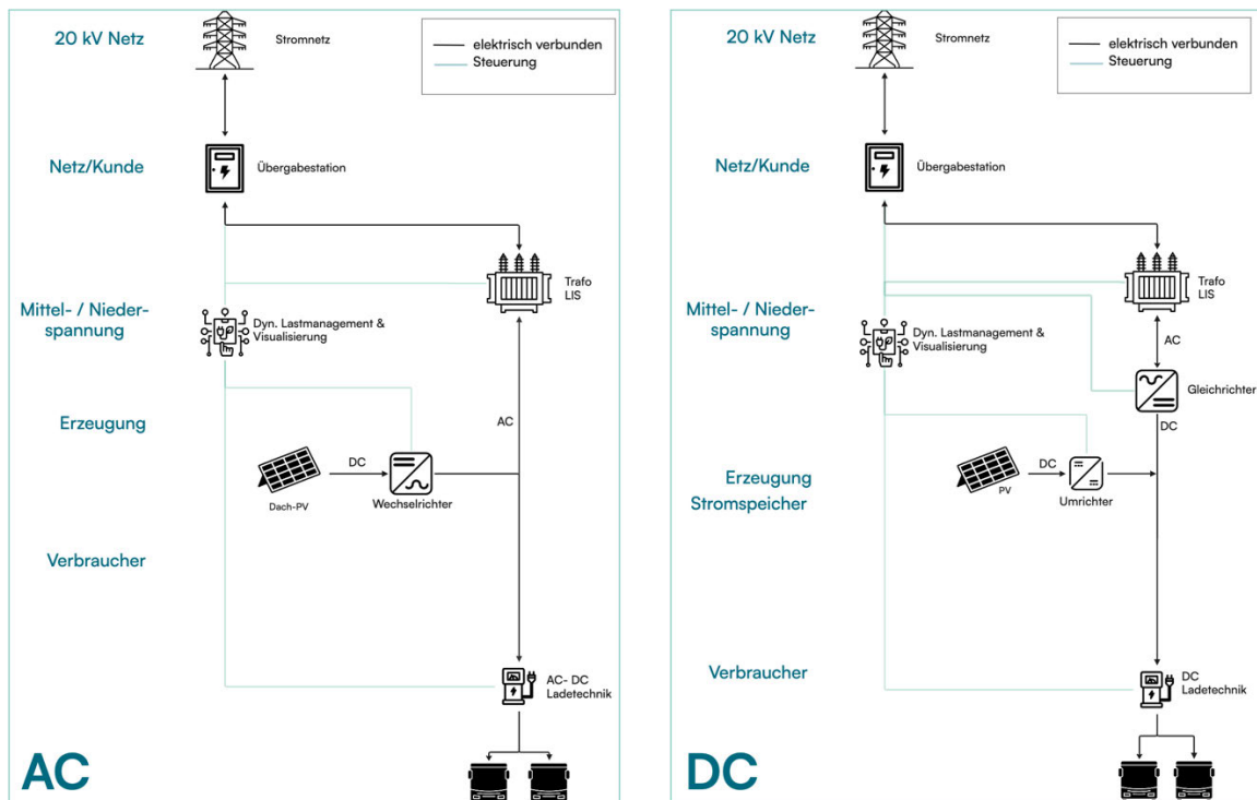
Abbildung 21: Schematische Darstellung des Energiesystems der Variante 3
