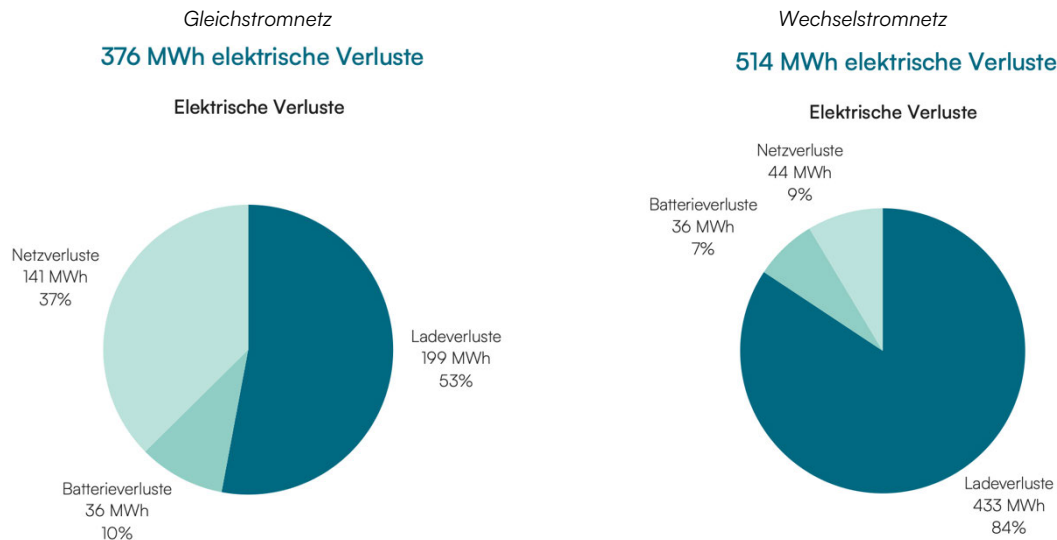
Abbildung 50: Gegenüberstellung der elektrischen Verluste - links DC-Netz und rechts AC-Netz — Variante 4 (Stufe 2)
