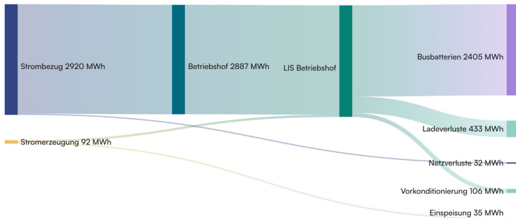
Abbildung 47: Elektrischer Energiefluss für Ausbaustufe 2 — Variante 3 mit reinem Strombezug
