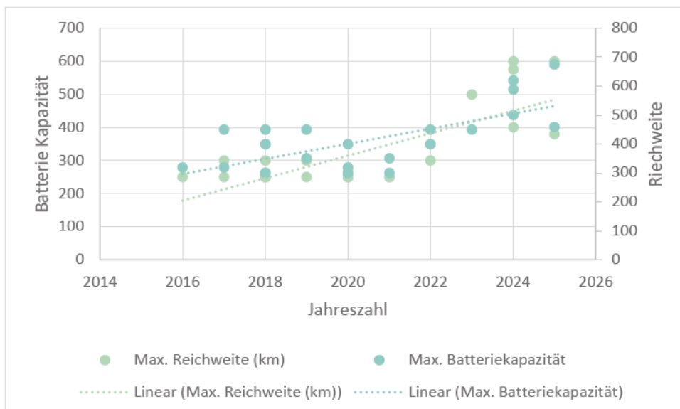
Abbildung 17: Kapazitäts- und Reichweitenentwicklung von Omnibussen
