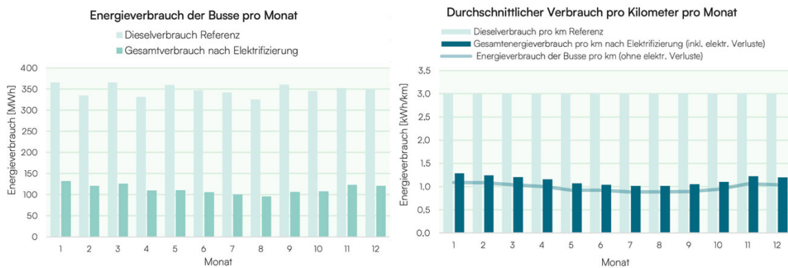
Abbildung 30: Vergleich des Energieverbrauchs - E-Bus vs. Dieseldbus (Stufe 1)
