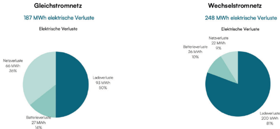
Abbildung 36: Gegenüberstellung der elektrischen Verluste - links DC-Netz und rechts AC-Netz — Variante 4 (Stufe 1)
