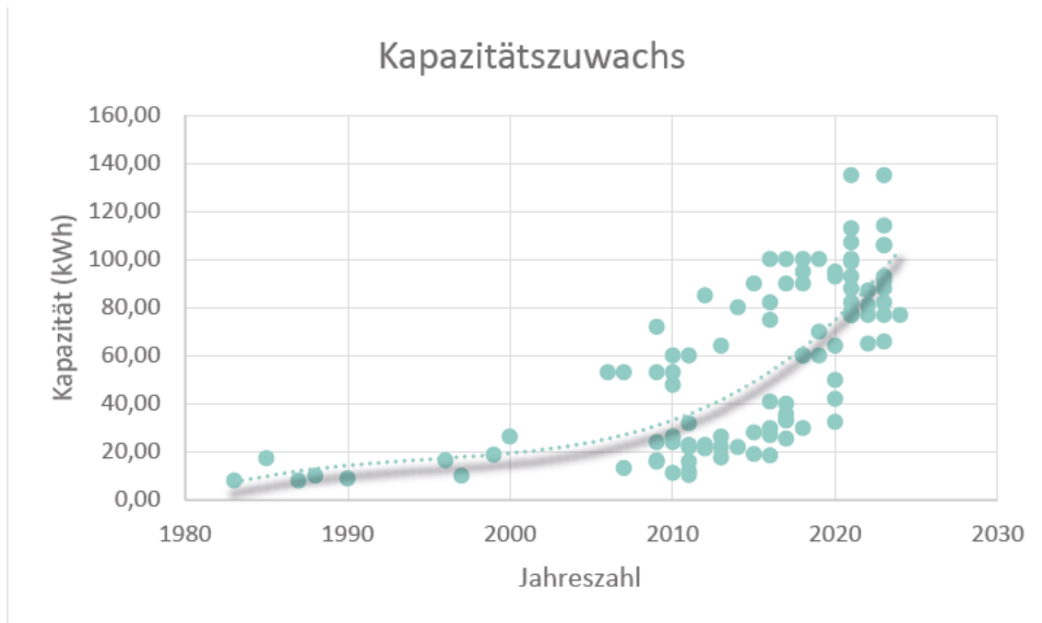
Abbildung 16: Batterieentwicklung; basierend auf den Werten von (Sanguesa et al. 2021).
