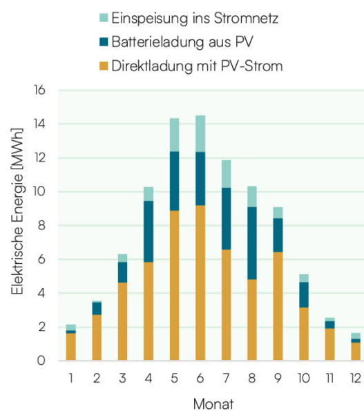
Abbildung 49: PV-Strom-Anteil am Energieverbrauch und Verhältnis von Eigennutzung und Einspeisung (Stufe 2, Variante 4)
