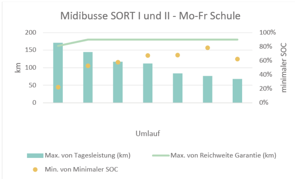
Abbildung 11: Midibusse SORT I und II (Schule) — Istzustands-Auswertung
