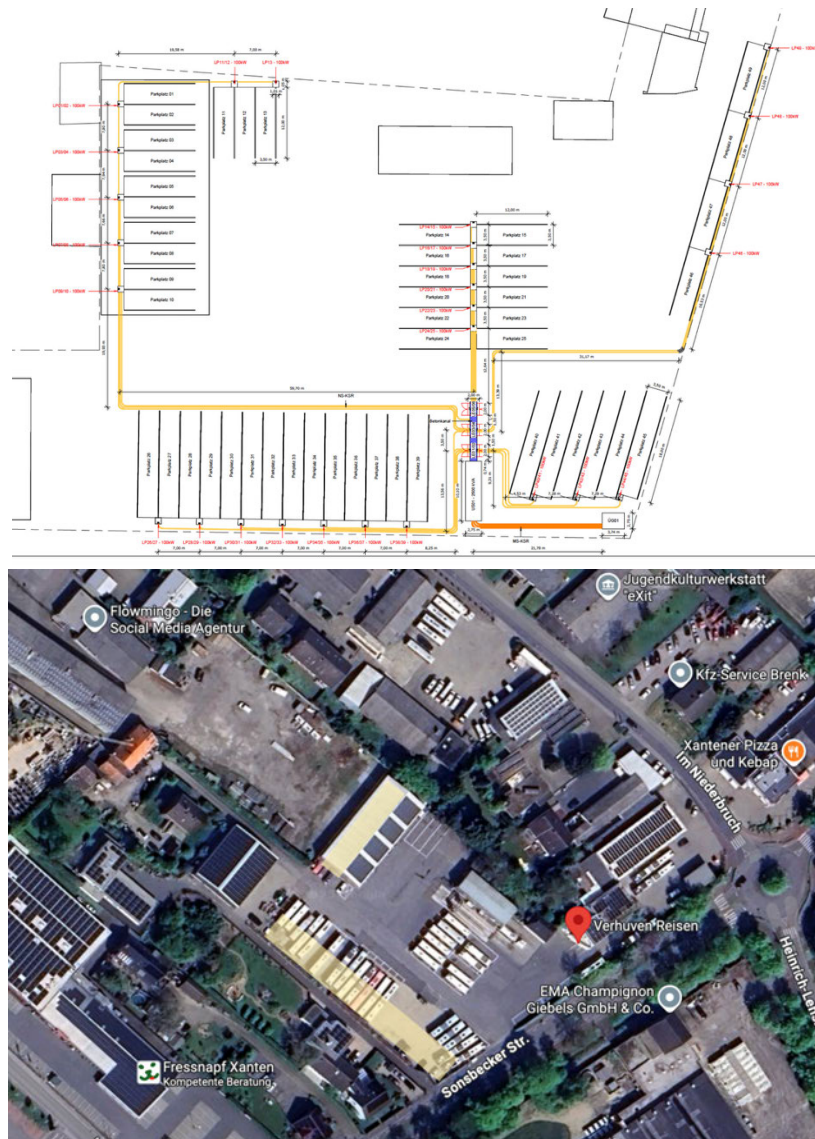
Abbildung 18: Mögliche PV-Fläche und zusätzliche Aufstellorte für Ladepunkte am Betriebshof
