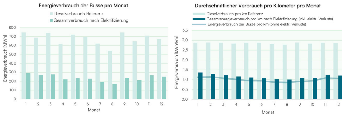
Abbildung 46: Vergleich des Energieverbrauchs - E-Bus vs. Dieselbus (Stufe 2 - Variante 3)
